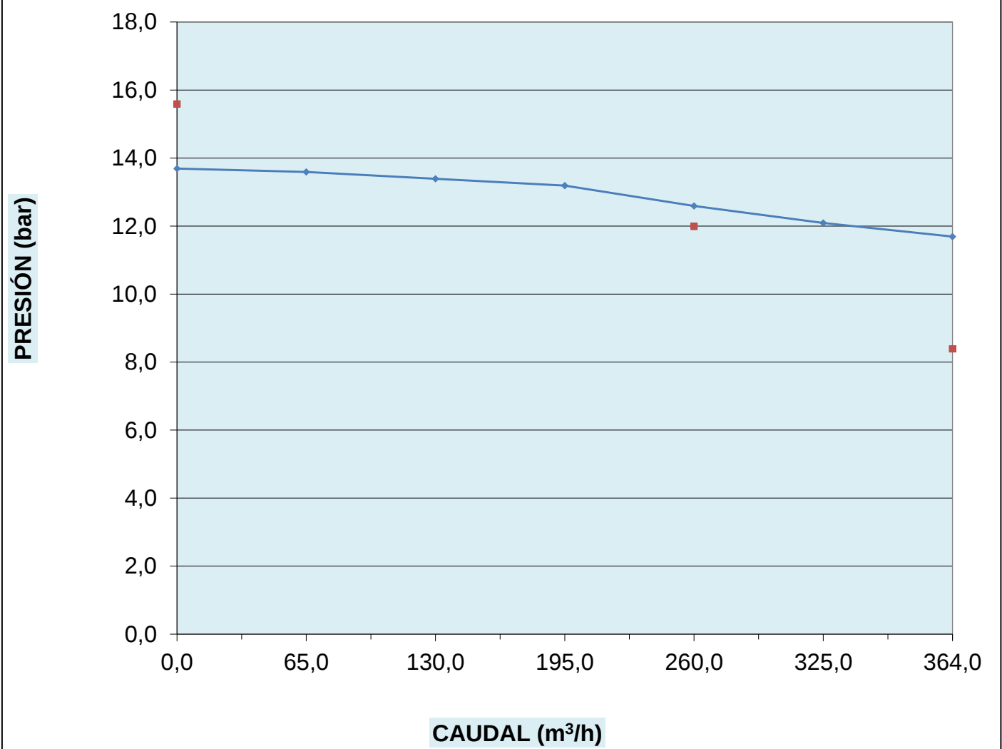
CURVA CAUDAL PRESIÓN BOMBA ELÉCTRICA 1
