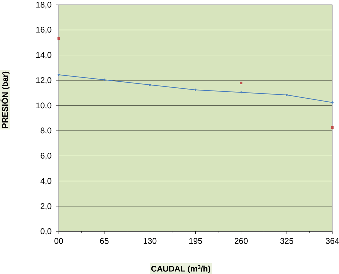
CURVA CAUDAL PRESIÓN BOMBA DIESEL 2
