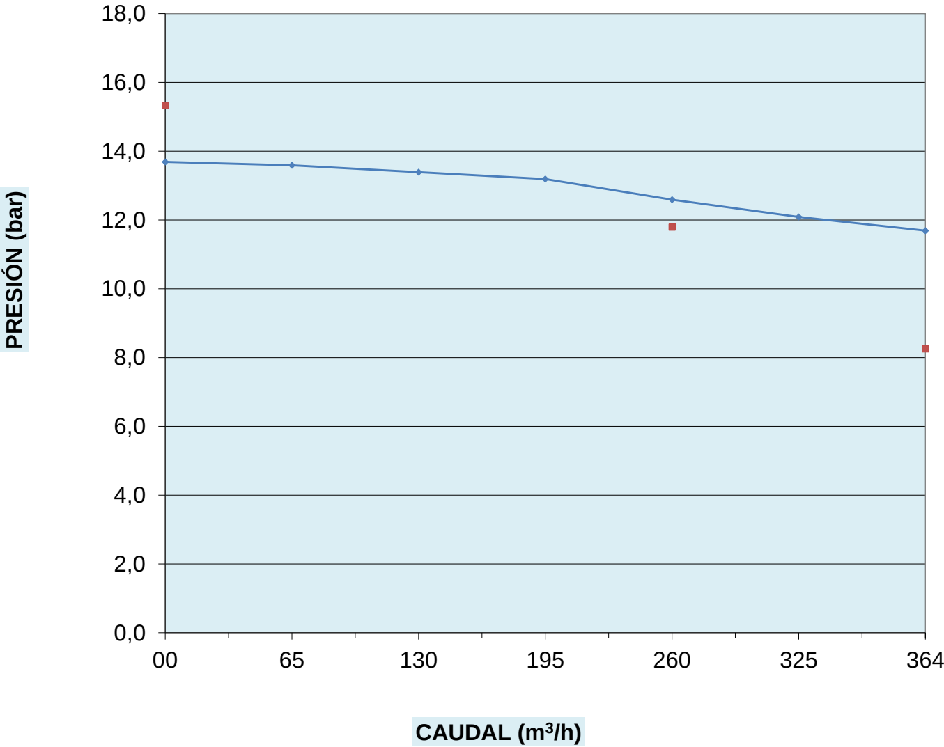
CURVA CAUDAL PRESIÓN BOMBA ELÉCTRICA 1
